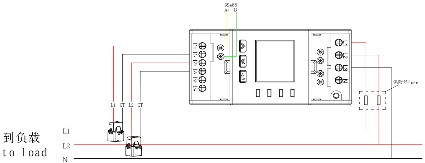
图 7 ADL400N-CT 单相三线经互感器接入
