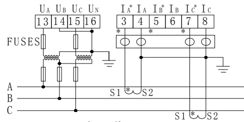
三相三线 2PT、2CT Three-phase 3-wire 2PT, 2CT
